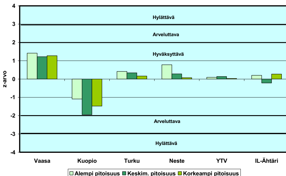
Kuva 13. Z-arvot otsonivertailussa.
