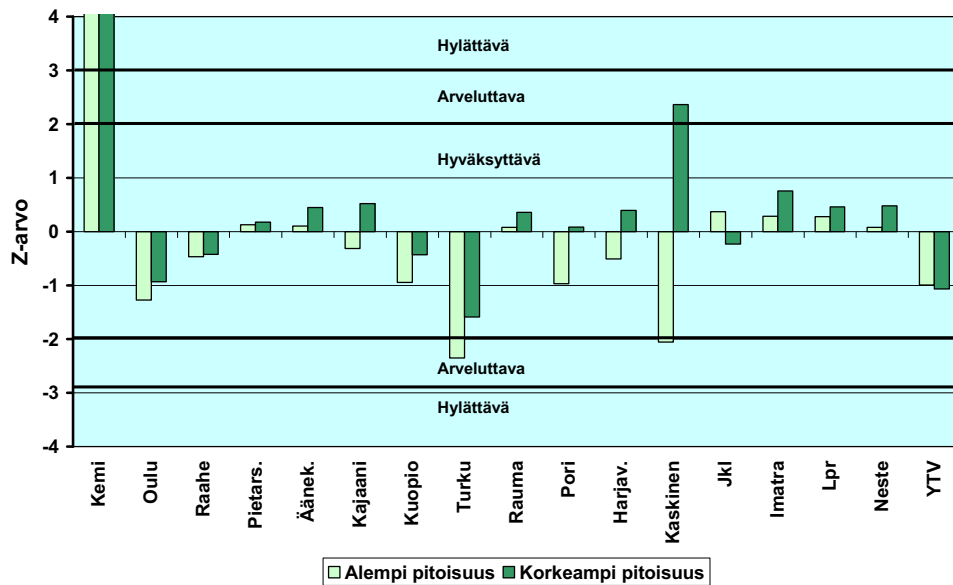
Kuva 10. Z-arvot rikkidioksidivertailussa.
