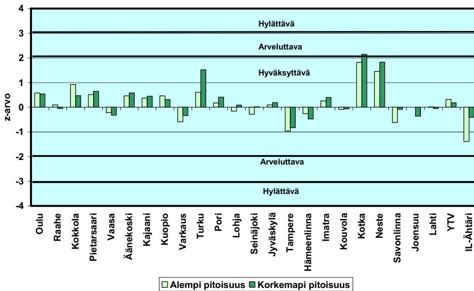
Kuva 11. Z-arvot typpimonoksidivertailussa.
