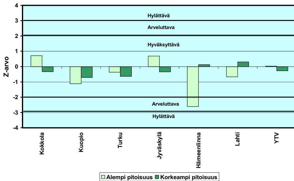
Kuva 9. Z-arvot hiilimonoksidivertailussa.
